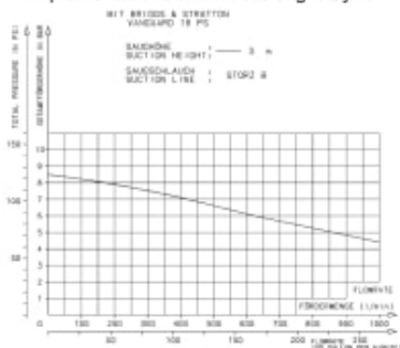
Kapasitetskurve Otter - 3m sugehøyde
